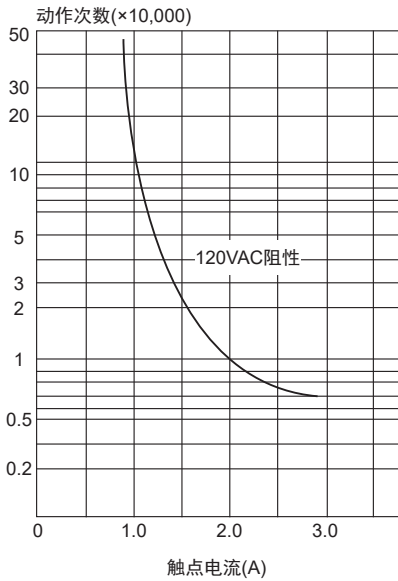
寿命曲线
