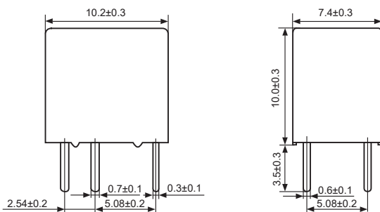
外形图
