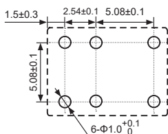
安装孔尺寸 (底视图)
