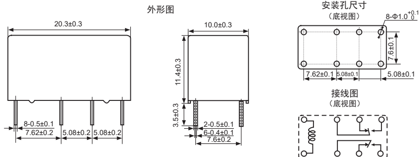
外形图、接线图、安装孔尺寸(单位:mm)
