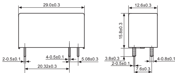
外形图
