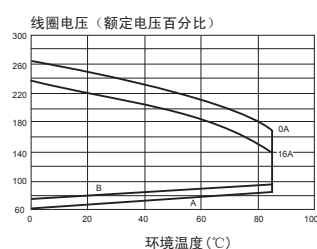
线圈工作范围曲线
