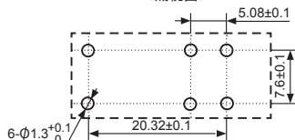
接线图 (底视图)
