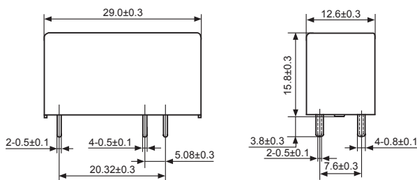
外形图
