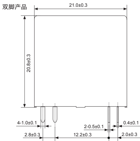
外形图
