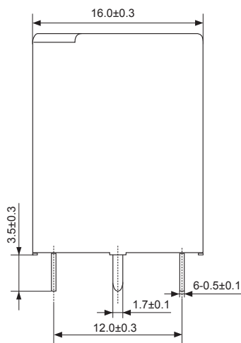
外形图
