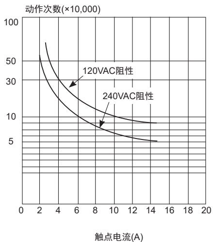
寿命曲线
