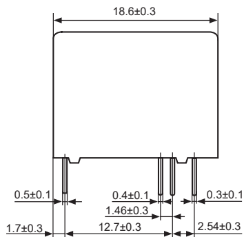
外形图
