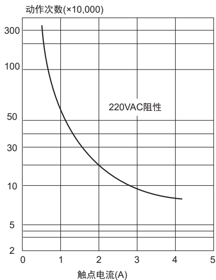
寿命曲线
