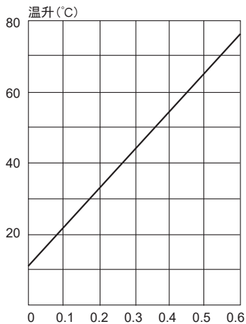
线圈温升
