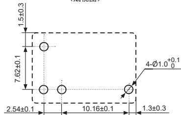
安装孔尺寸 (底视图)
